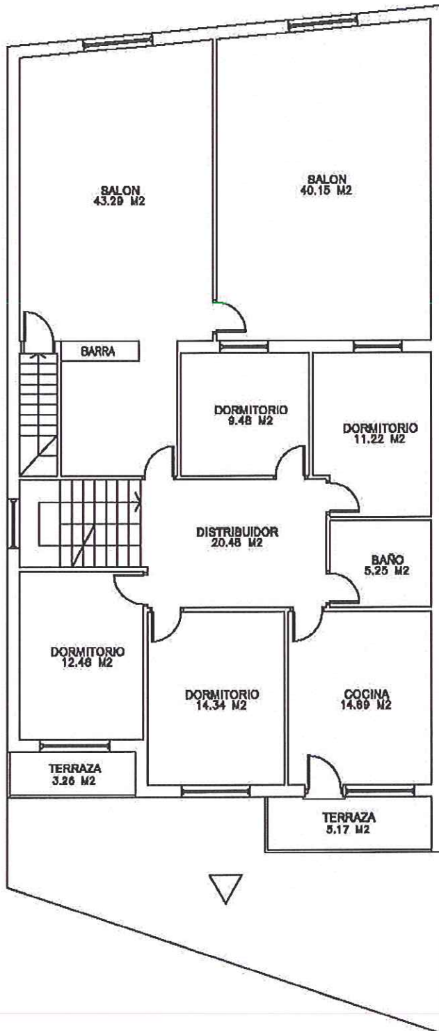
PLANTA PRIMERA
